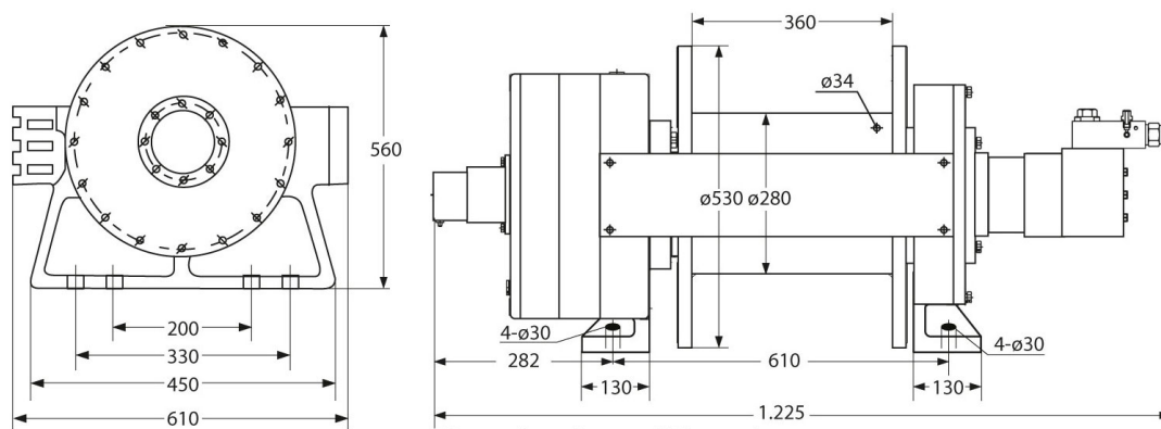
Dimensions in mm / Dimensiones en mm
