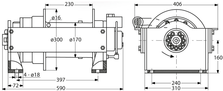
Dimensions in mm / Dimensiones en mm Imágenes Referenciales
