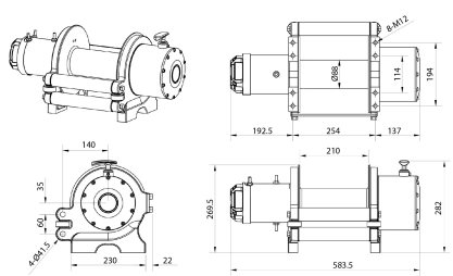
Dimensions in mm / Dimensiones en mm
