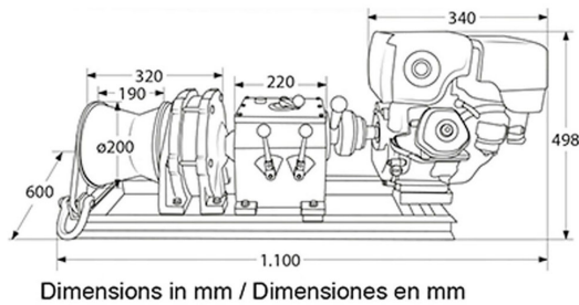
Dimensions in mm / Dimensiones en mm
