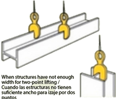
Vertical lifting of steel structures / Izaje vertical de estructuras de acero
