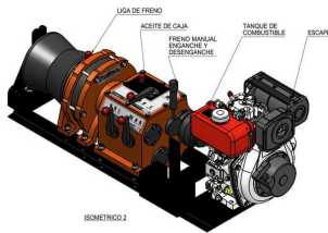
ISOMETRICO 2
