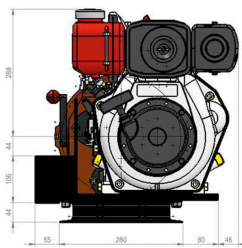
VISTA POSTERIOR
