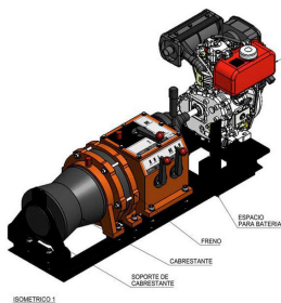
ISOMETRICO 1
